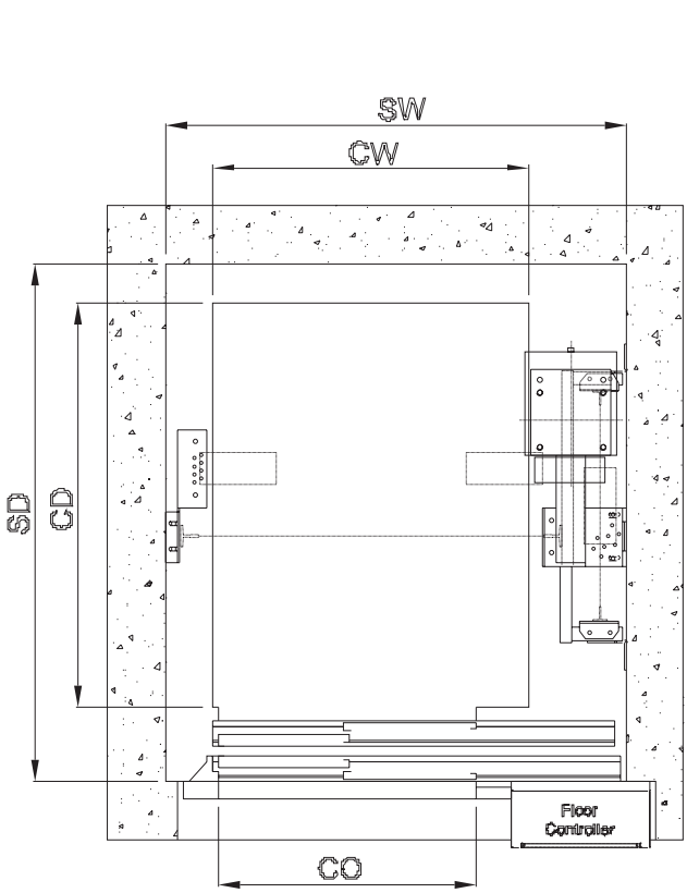
630 kg / 1 Side Opening Door
